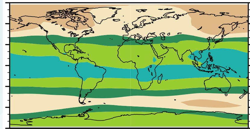
E3SM
